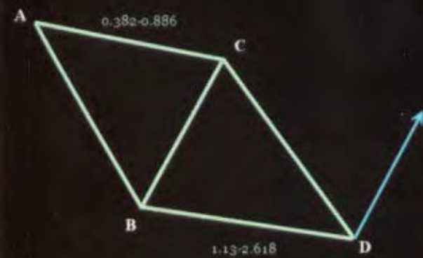
ABCD (Bullish)
