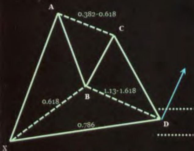
Gartley (Bullish)
